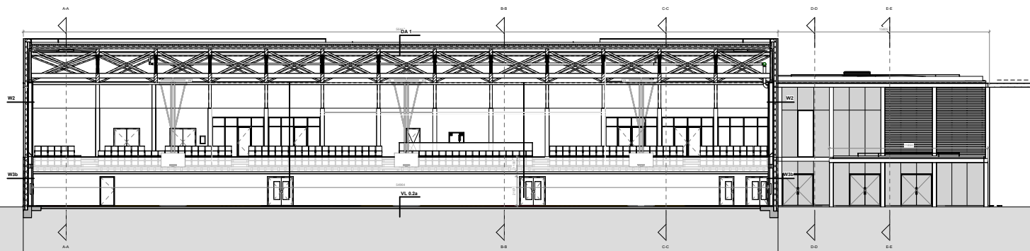
LANGSDOORSNEDE OVER DE GROTE SPORTHAL
