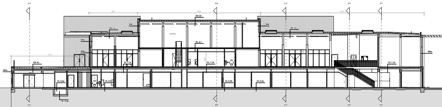
LANGSDOORSNEDE OVER DE MIDDENZONE EN INKOM
