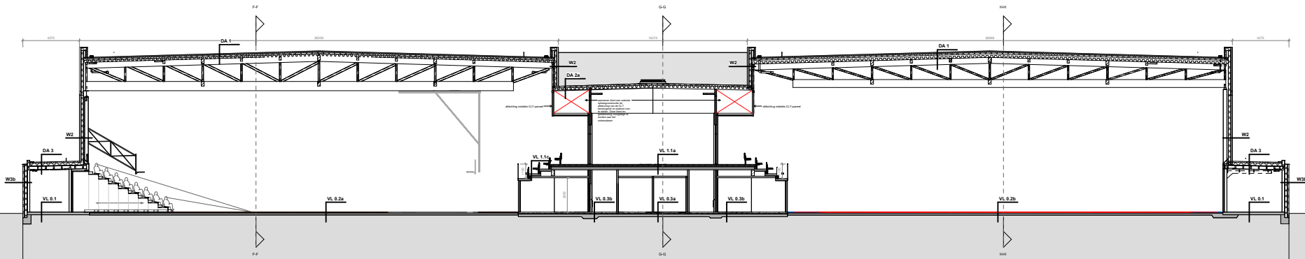
DWARSDOORSNEDE OVER DE HALLEN EN DE MIDDENZONE MET MULTIFUNCTIONLE RUIJITE
