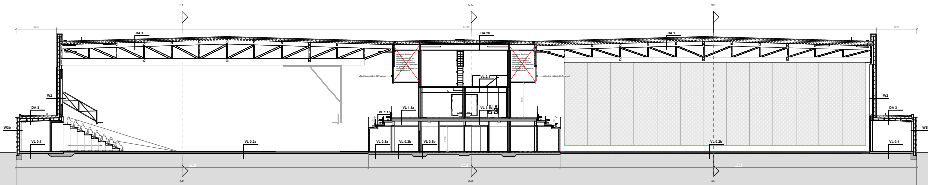
DWARSDOORSNEDE OVER DE HALLEN EN DE MIDDENZONE MET TECHIEKRUIJITE
